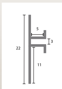
Offenes H- Profil
