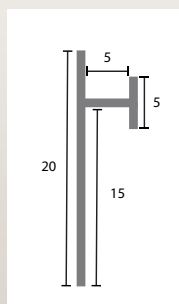
H- Profil
